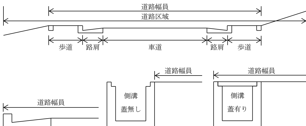
図1 道路幅員
