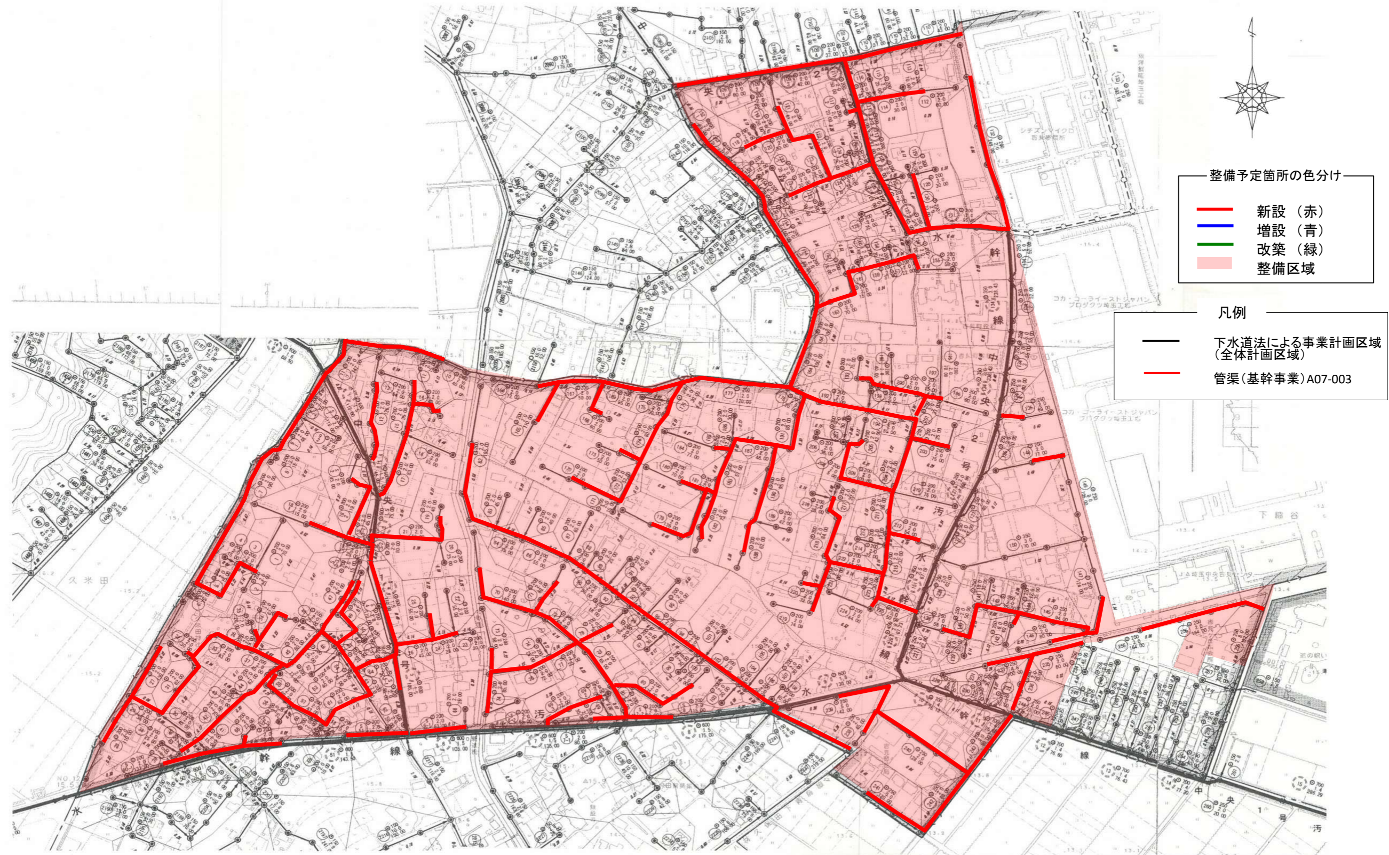
吉見町下水道事業 管渠整備 中央地区(未普及解消) 計画図
