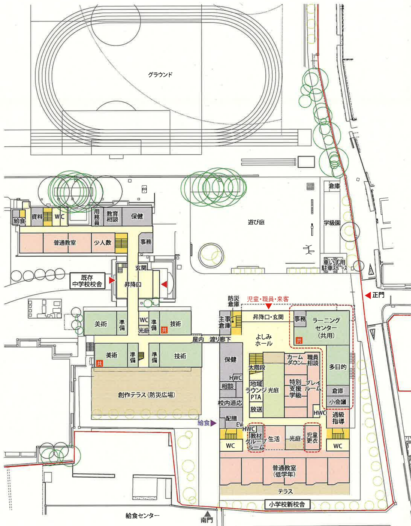
1 階平面図
