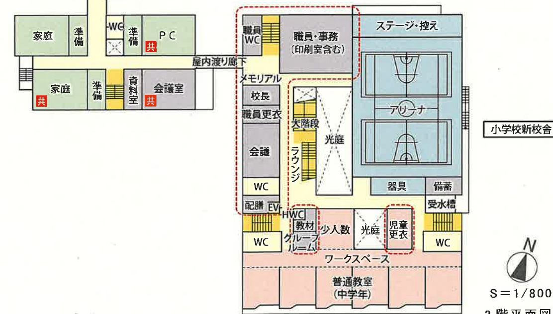
2 階平面図
