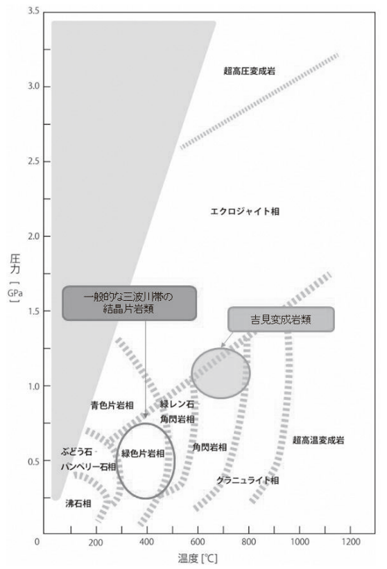
▲グラフ「変成岩の変成条件」
