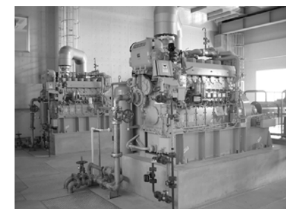
▲ポンプを移動するディーゼルエンジン
