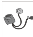
血圧測定
