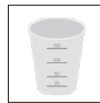
尿検査
