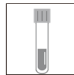
血液検査
