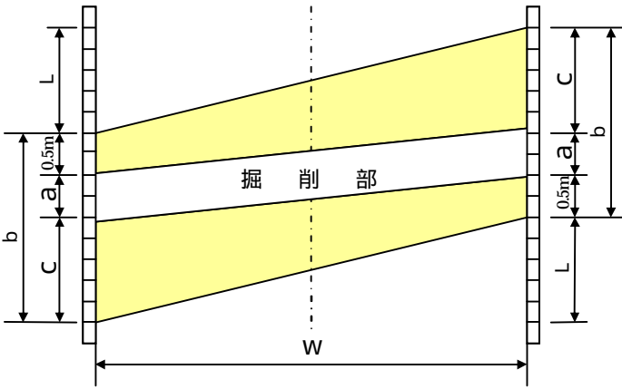
横断占用（斜横断）
